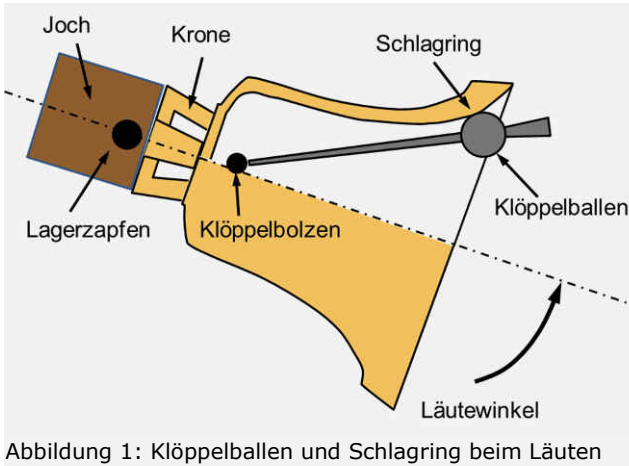
Abbildung 1: Klöppelballen und Schlagring beim Läuten
